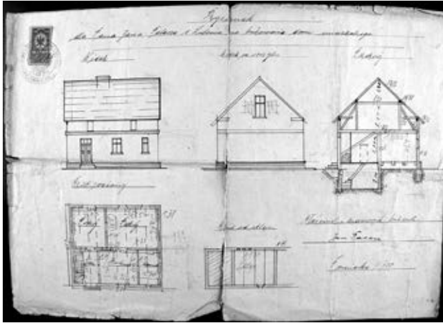
Rysunek domu budowanego przy ul. Narutowicza 7, którego właścicielem i kierownikiem budowy był Jan Palacz. Pozwolenie na budowę uzyskano 18.07.1925 r., podpisane przez sołtysa Andrzeja Remleina
