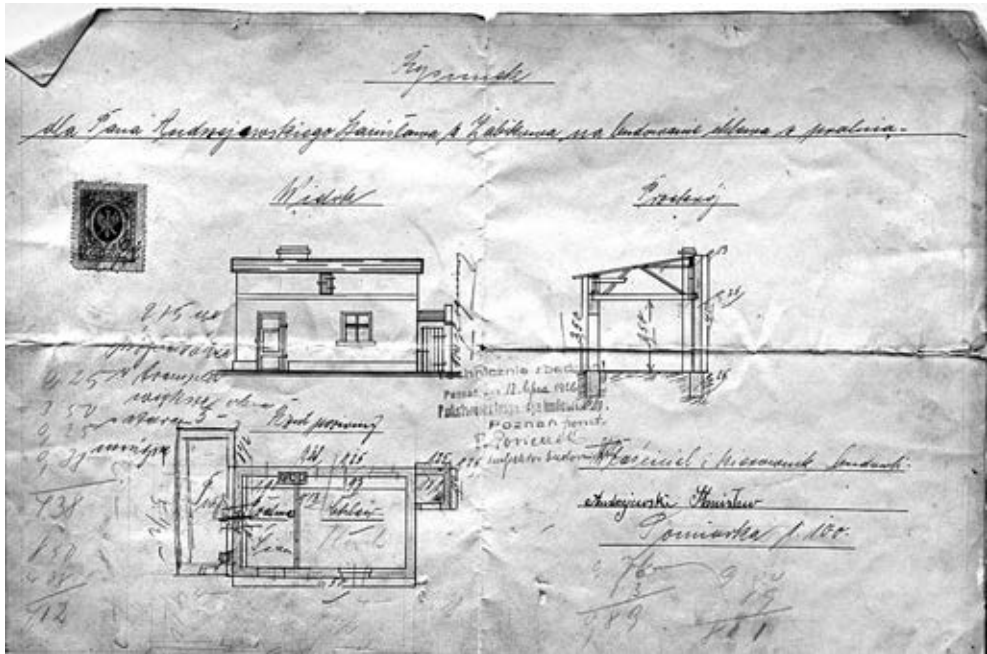
Plan domku robotnika Stanisława Andrzejewskiego, który w 1926 roku budował przy ul. Kościuszki 31
